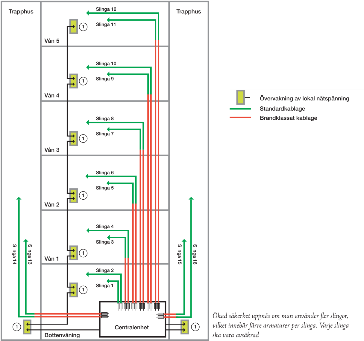
Exempel på kabelförläggning vid flera brandceller.
