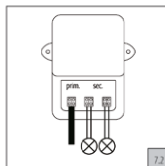
Två armaturer 2x200W/30V
